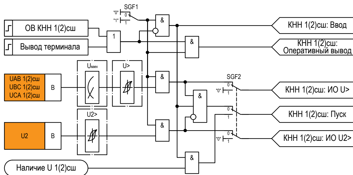
Рисунок 2.37 – Функциональная схема логики функции «КНН 1(2)сш»
